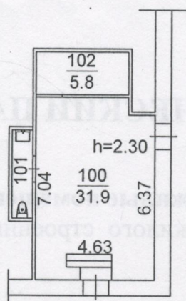
План помещений подвала
